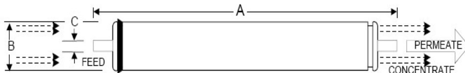
膜元件尺寸**
